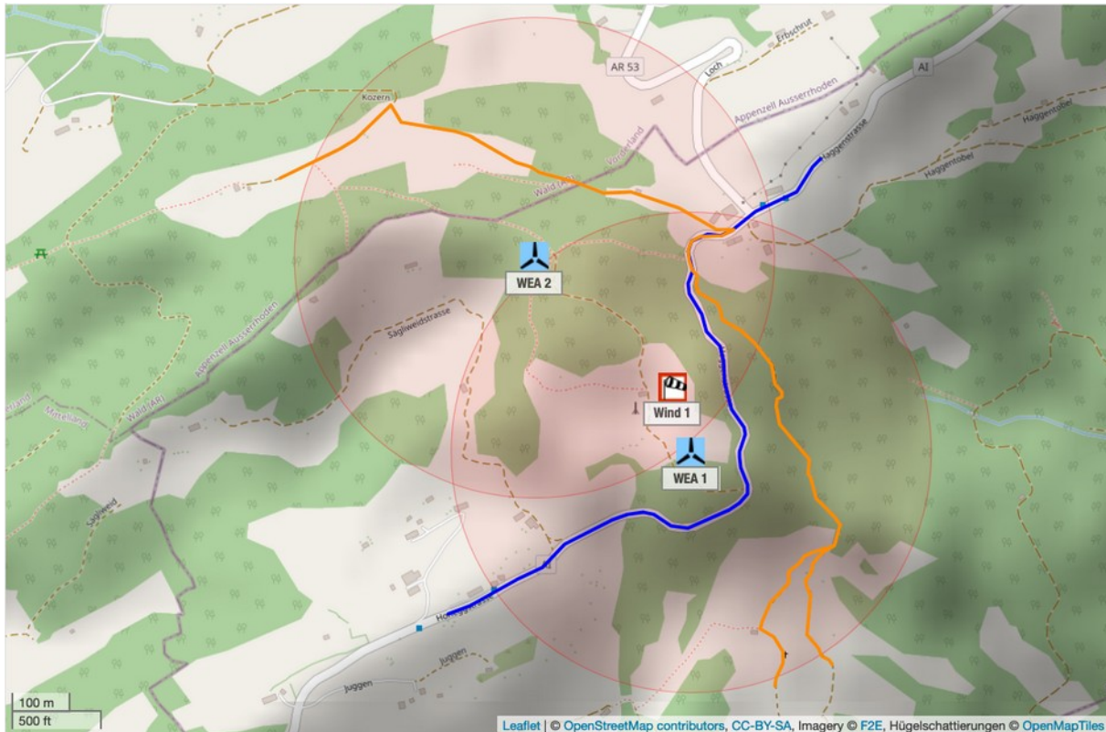
Abbildung 4.3.1: Potentielle Gefährdungsbereiche der WEA 1 und 2 und Schutzobjekte am Standort Oberegg AI (Karte /1.4/).
