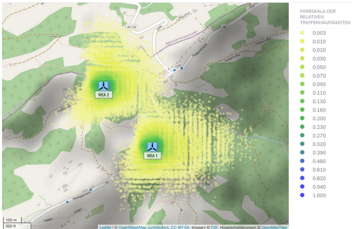
Abbildung A.1.1: Trefferhäufigkeiten von Eisstücken pro Rasterfläche ( 16m^2 ) und Jahr in der Umgebung der WEA 1 und 2 am Standort Oberegg AI (Karte /1.4/).
