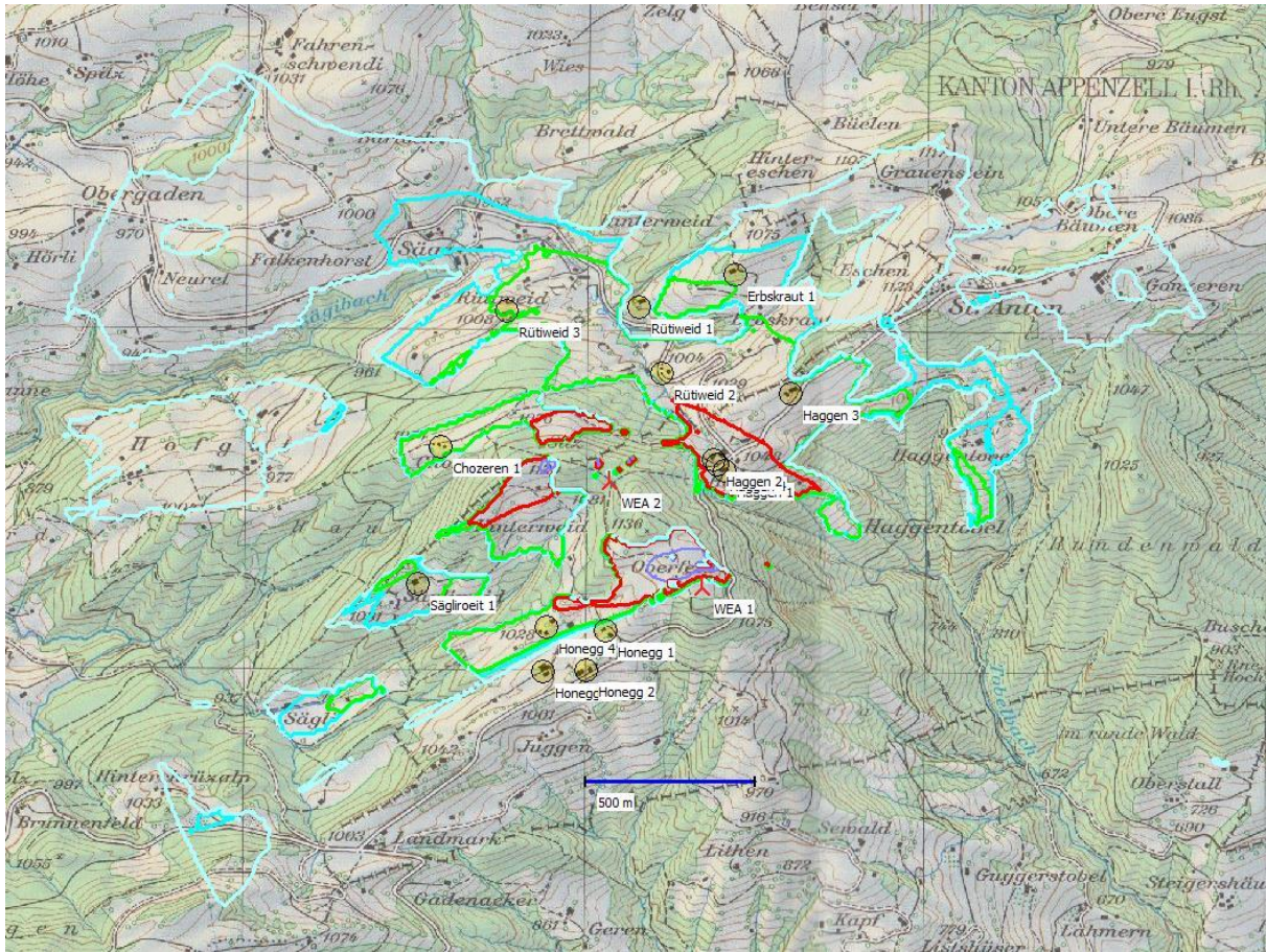
Abbildung 19: Meteorologisch wahrscheinliche Schattenwurfdauer in Stunden/Jahr (JH Wind)
