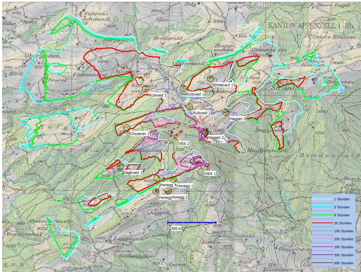
Abbildung 18: Astronomisch maximal mögliche Schattenwurfdauer in Stunden/Jahr. (Quelle: JH Wind)
